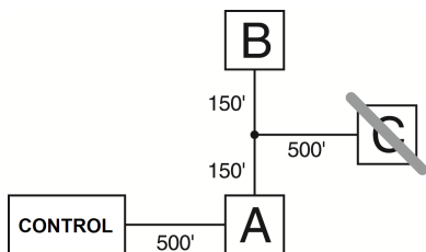
Figura 1-1 Cableado Corbus
