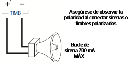
Figura 1-5 Cableado de terminales sirena
