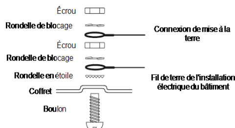
Figure 1-7 Mise à la terre
