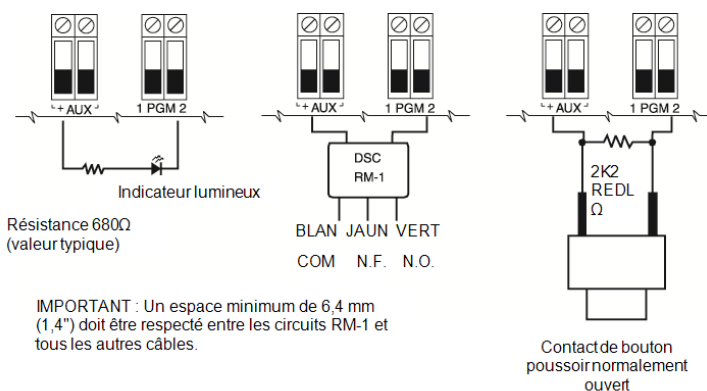
Figure 1-2 Sortie de voyant à résistance de limitation de courant et sortie à étage de relais facultative.
