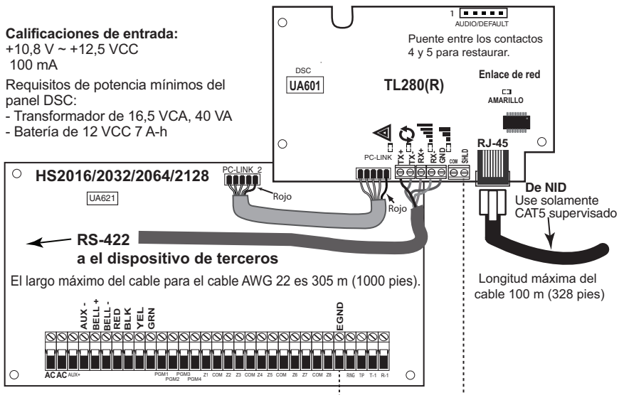
Figura 3: Diagrama de cableado del Comunicador
