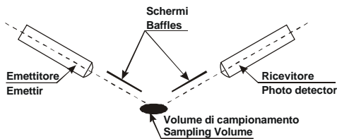
Fig. 1 Schema di funzionamento del sensore - System schematic
