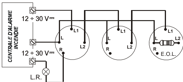
Fig. 2 Principe Câblage
