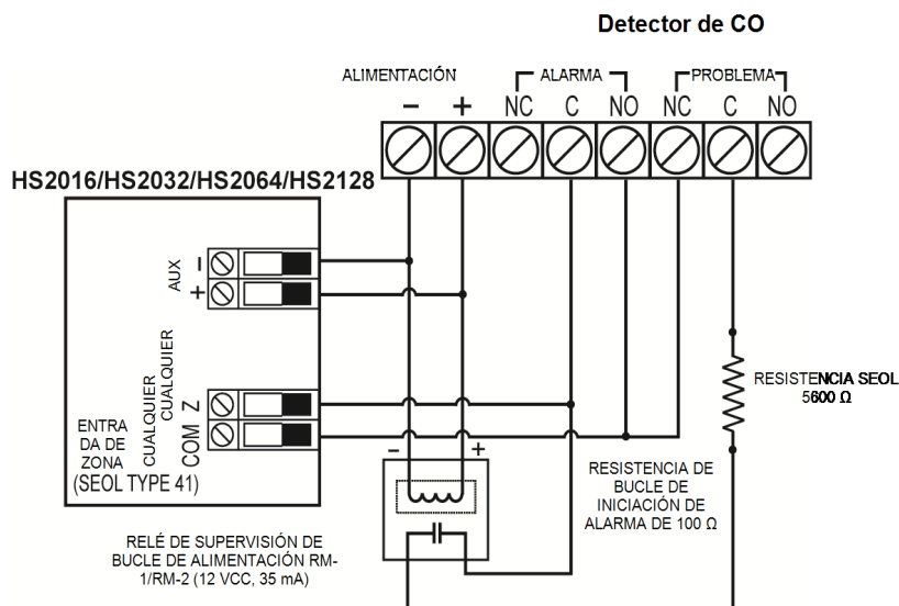
Figura 3-14 Cableado del detector de CO
