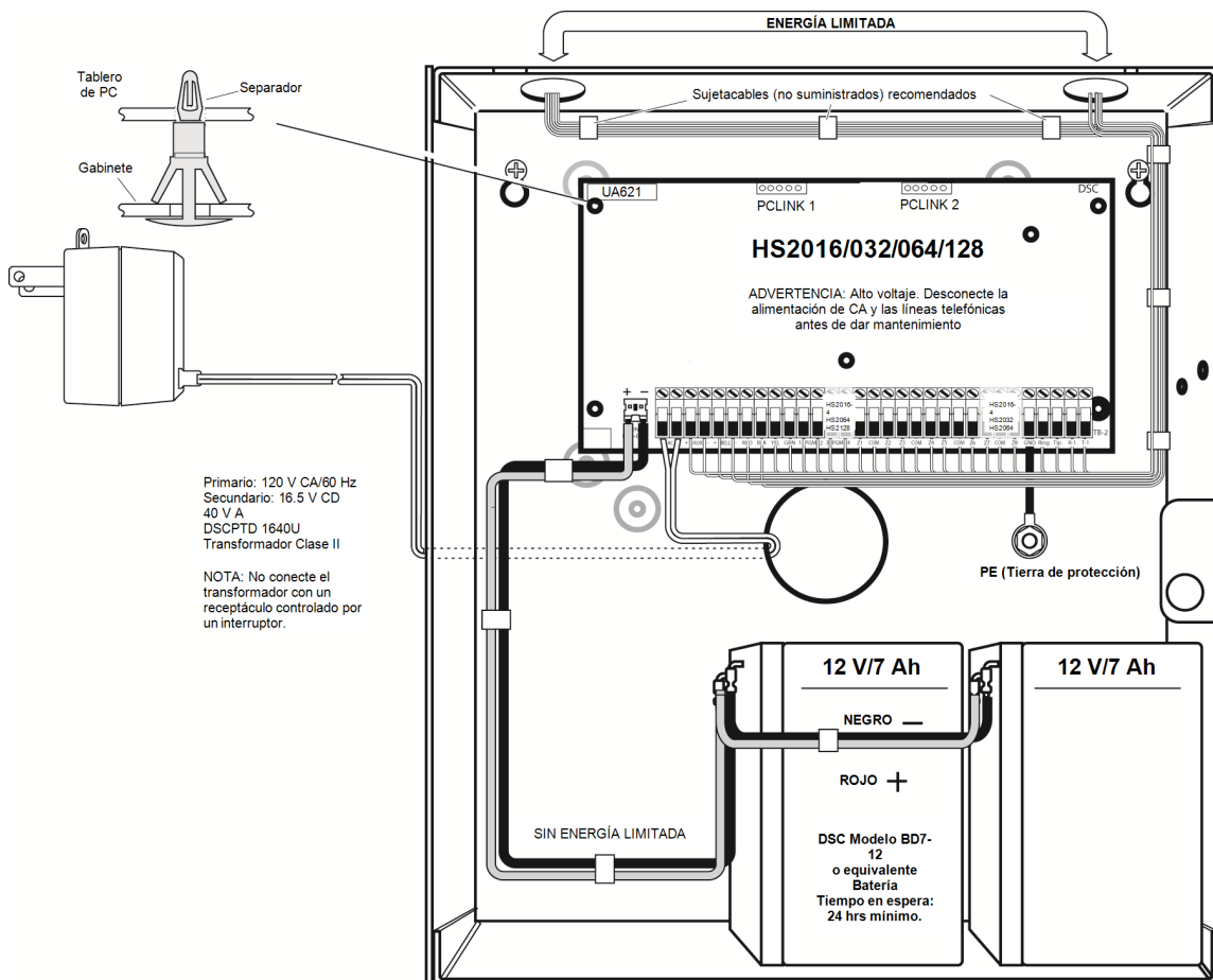
Figura 2-1 Enrutamiento de cableado (América del Norte solamente)
