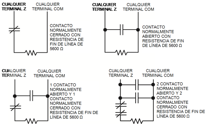
Figura 3-7 Cableado de SEOL
