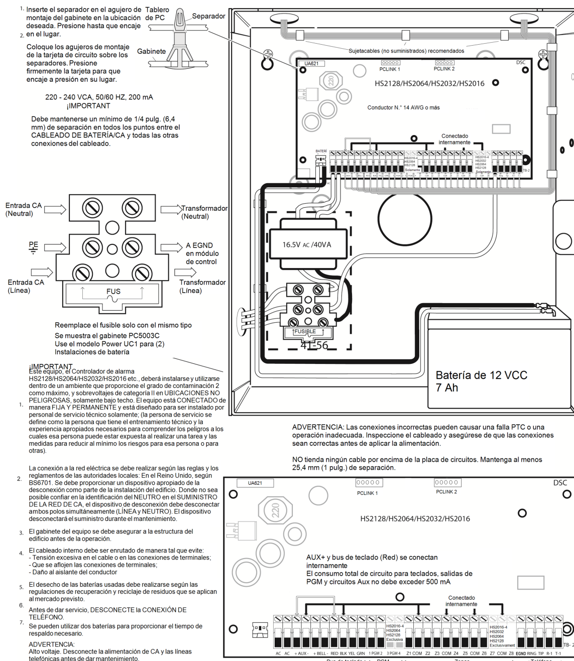
Figura 2-2 Enrutamiento de cableado (exclusivo para EN50131)
