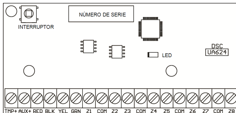
Figura 3-1 HSM2108 Expansor de zona
