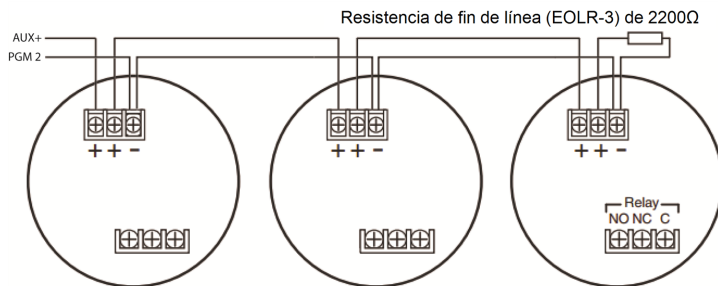
Figura 3-13 Cableado de detector de humos de dos hilos
