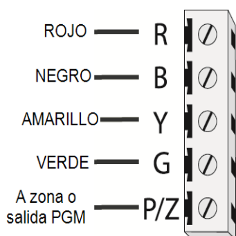
Figura 3-5 Terminales P/Z del teclado
