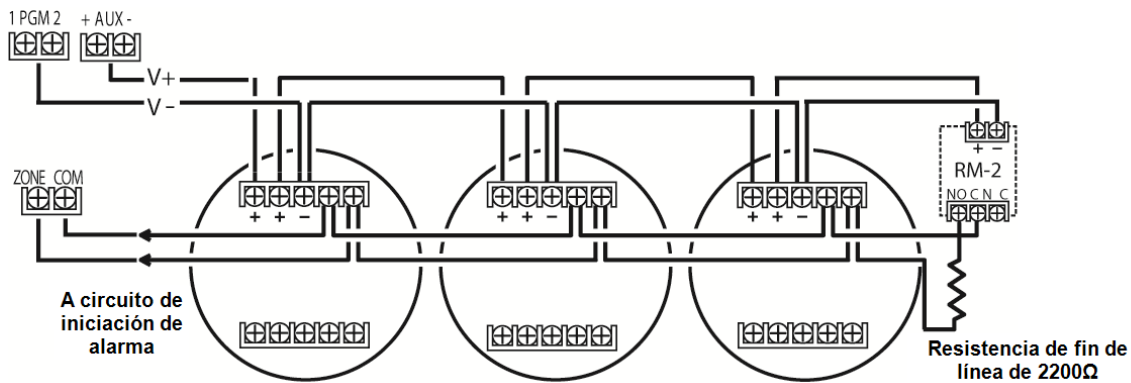
Figura 3-12 Cableado del detector de humo
