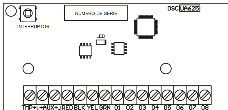
Figura 3-2 HSM2208 Expansor de salida
