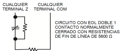
Figura 3-8 Cableado de DEOL
