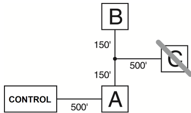
Figura 2-3 Cableado Corbus
