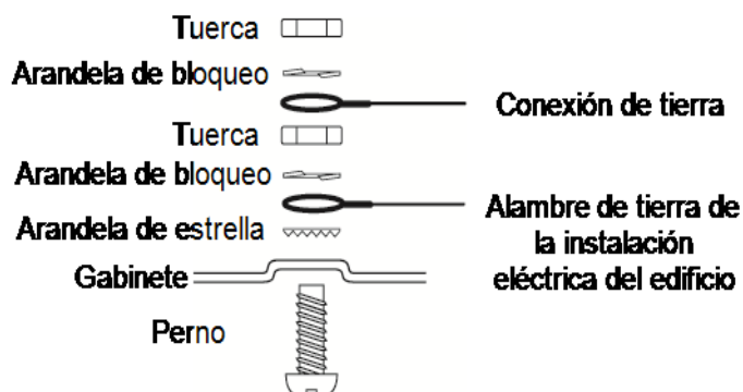
Figura 3-15 Instalación de tierra
