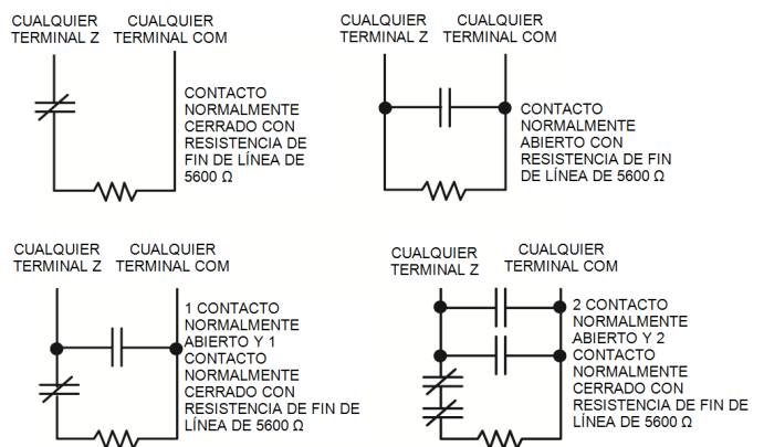
Figura 1-3 Cableado de SEOL
