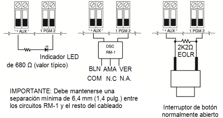
Figura 1-2 Salida LED con resistencia limitadora de corriente y salida opcional de controlador de relé.
