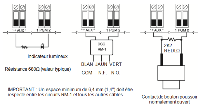
Figure 1-2 Sortie de voyant à résistance de limitation de courant et sortie à étage de relais facultative.
