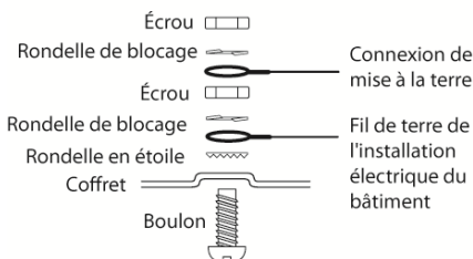
Figure 1-7 Mise à la terre
