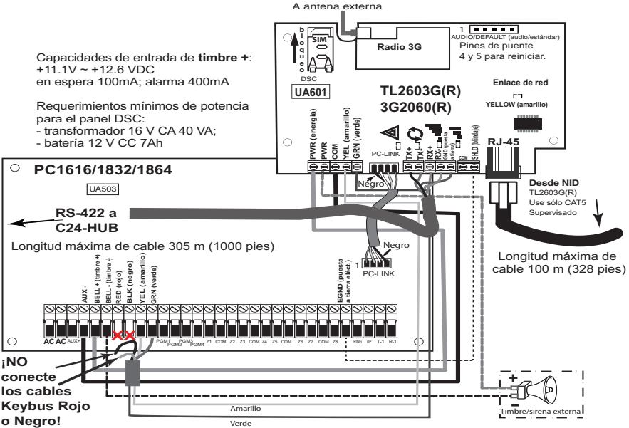
Figure 3: Diagrama de cableado del Comunicador
